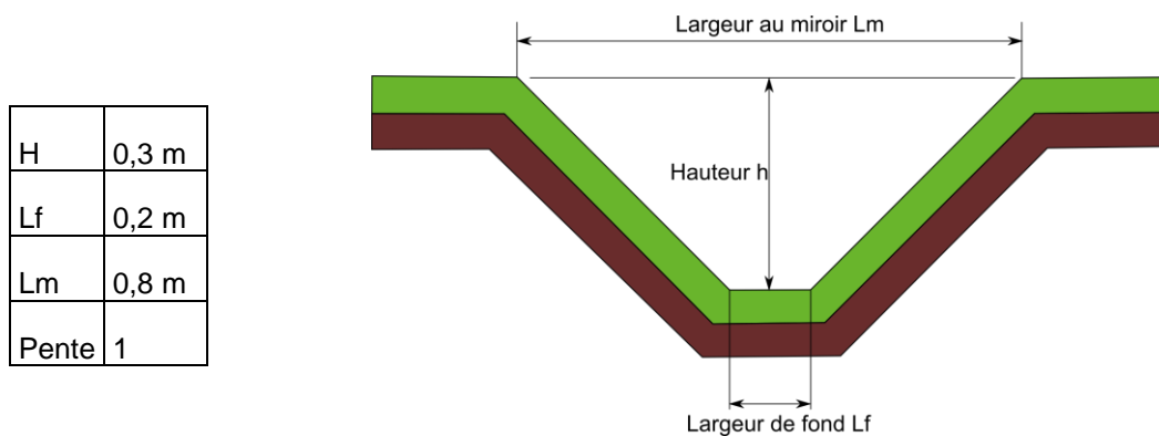
Fig. 27. Coupe type du fossé à mettre en place – Chemin Malefosse
